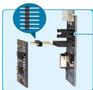
数传模块TTL接口连接示意图
